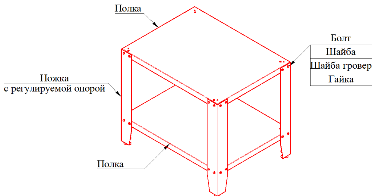
Рис. 1 - Схема сборки подставки. Подставка поставляется в разобранном виде.
