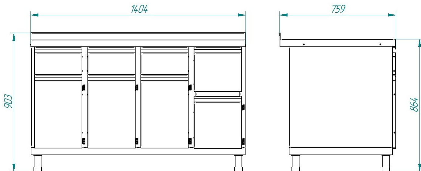
Рис.1 Общий вид СКМ-7-2
