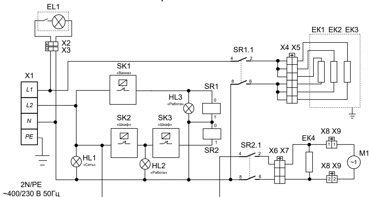
Схема электрическая ЭМК-70КМШ
