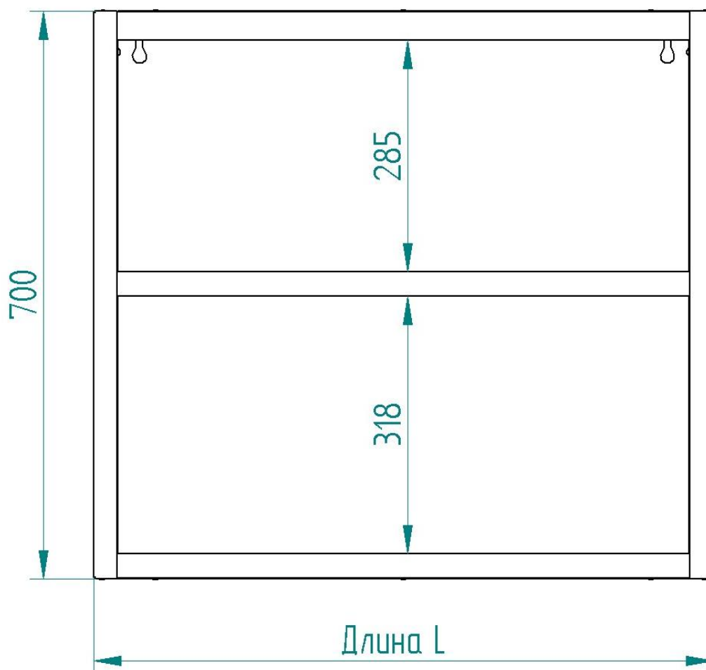
Рис. 3 Полка ПНО (вид спереди)
