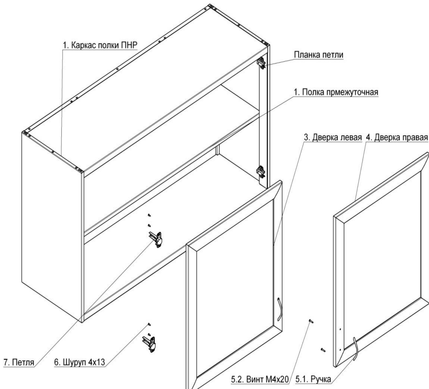
Рисунок 2. Схема для сборки полки типа ПНР.
