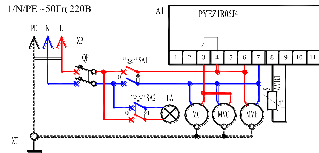
Рис.4. Схема электрическая принципиальная шкафа холодильного Carboma R1400K.
